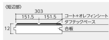
■断面図 (単位mm)
